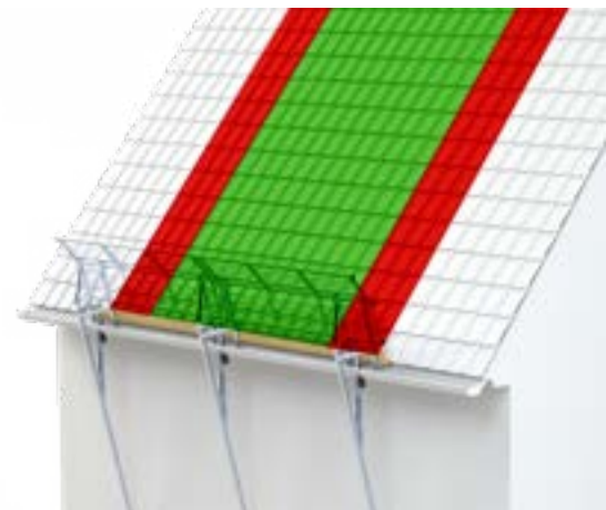
toegestaan werkgebied
